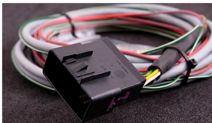
Fig 1b - Medföljande extra kabelhärva(10) med monterat kontaktdon för inkoppling av MaxxECUs medföljande bredbandslambdasond. Monteras och klipps till rätt längd beroende på vart lambdasonden placeras.
